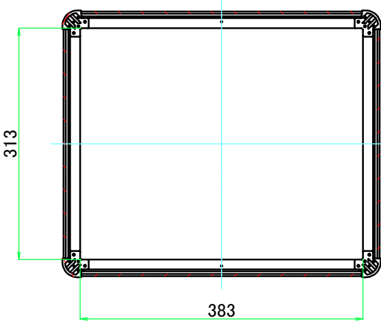
C-C ( 1 : 7 )
